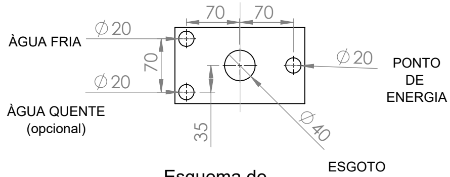
Esquema de instalação (Sob acento)
